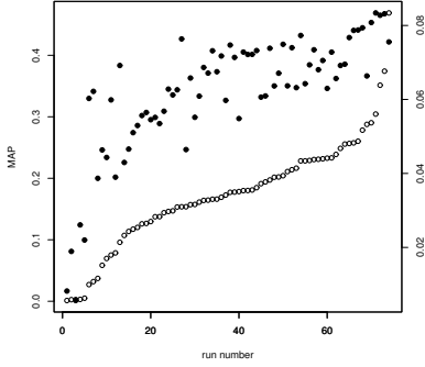
(d) TREC-6 ( \tau = 0.635 )
